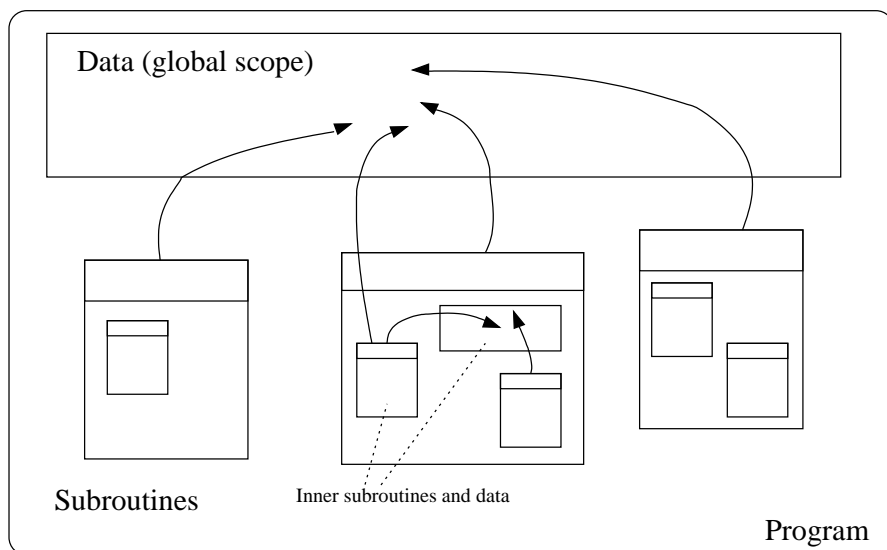
Рис. 1.2: Топология языков программирования конца второго и начала третьего поколения
