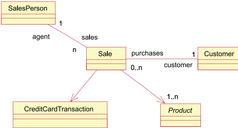
Рис. 4.3: Диаграмма классов торговой сделки.
